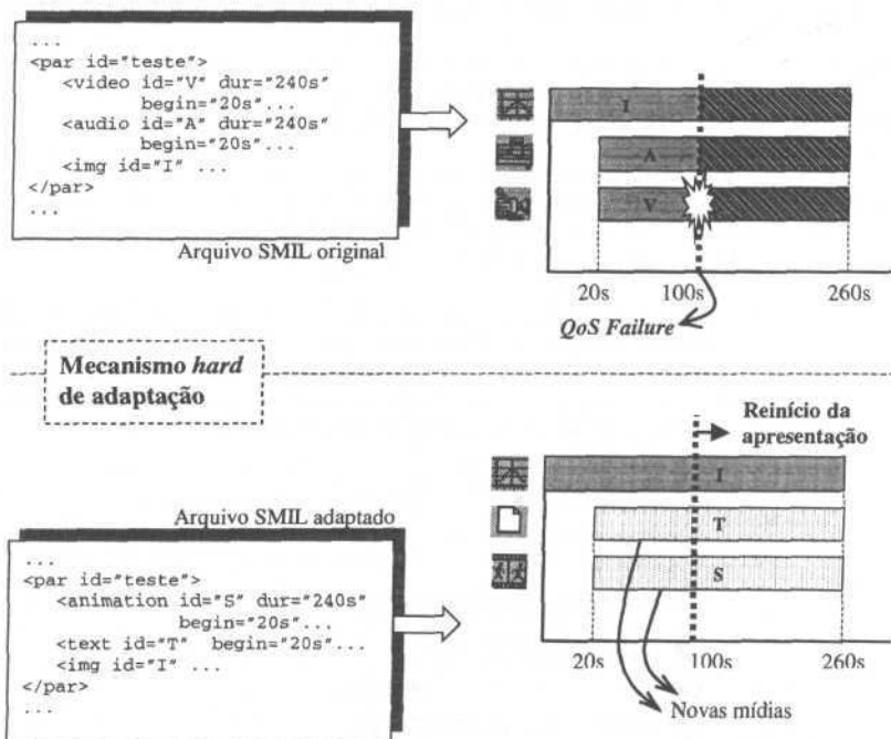
Figura 8- Adaptação hard
