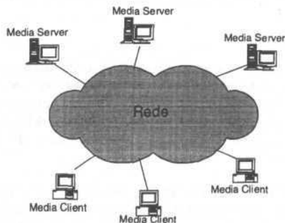
Figura 4- Ambiente Cliente-Servidor
