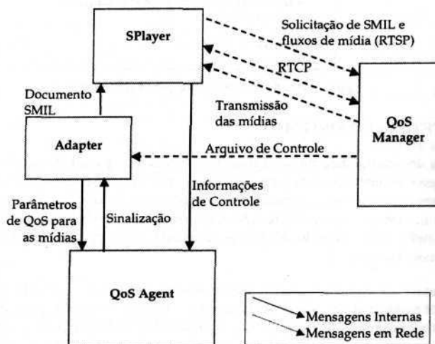
Figura 6- Esquema de comunicação entre os módulos
